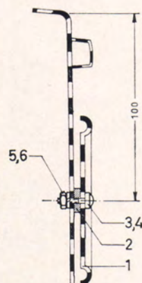
Schnitt A-B
