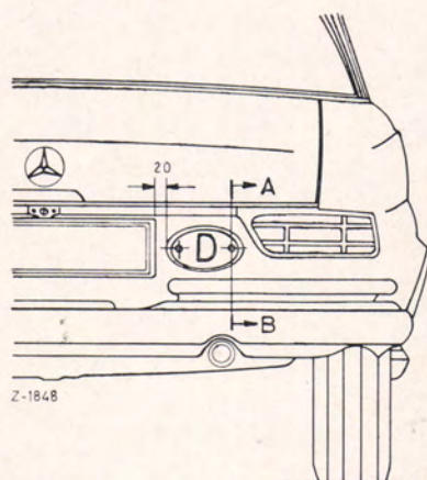
Schnitt A-B
